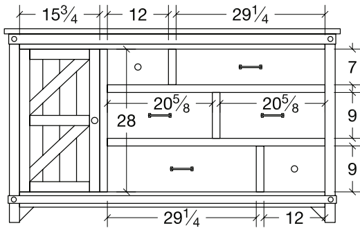
Door Dresser (CLDDR)
