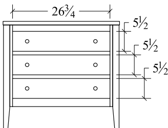
Nightstand (HENS332) 3 drawer 32w x 16d x 29 1/2h
